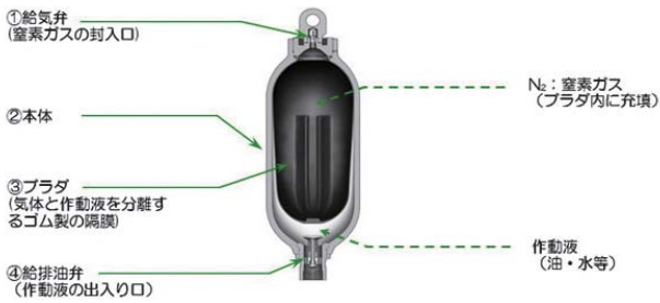
アキュムレータの構造
